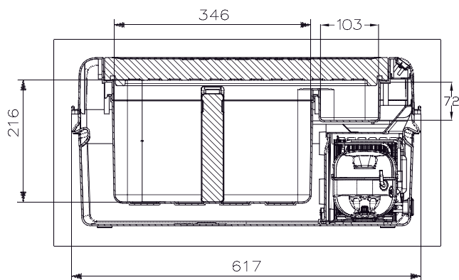
Схема AF-L20 ЛЕДЯНОЙ
