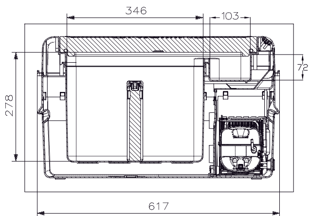
Схема AF-L25 ЛЕДЯНОЙ
